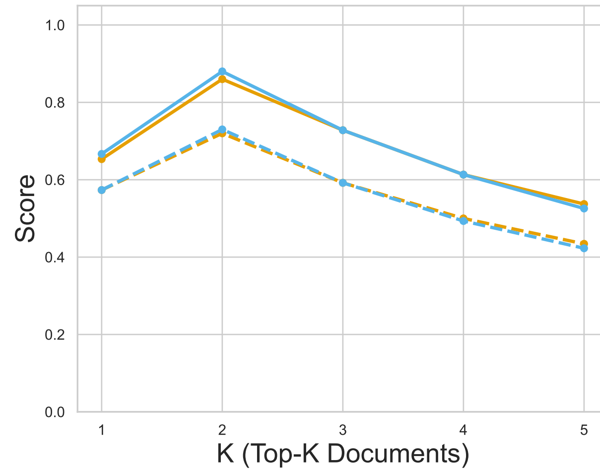
F1-Score@K
