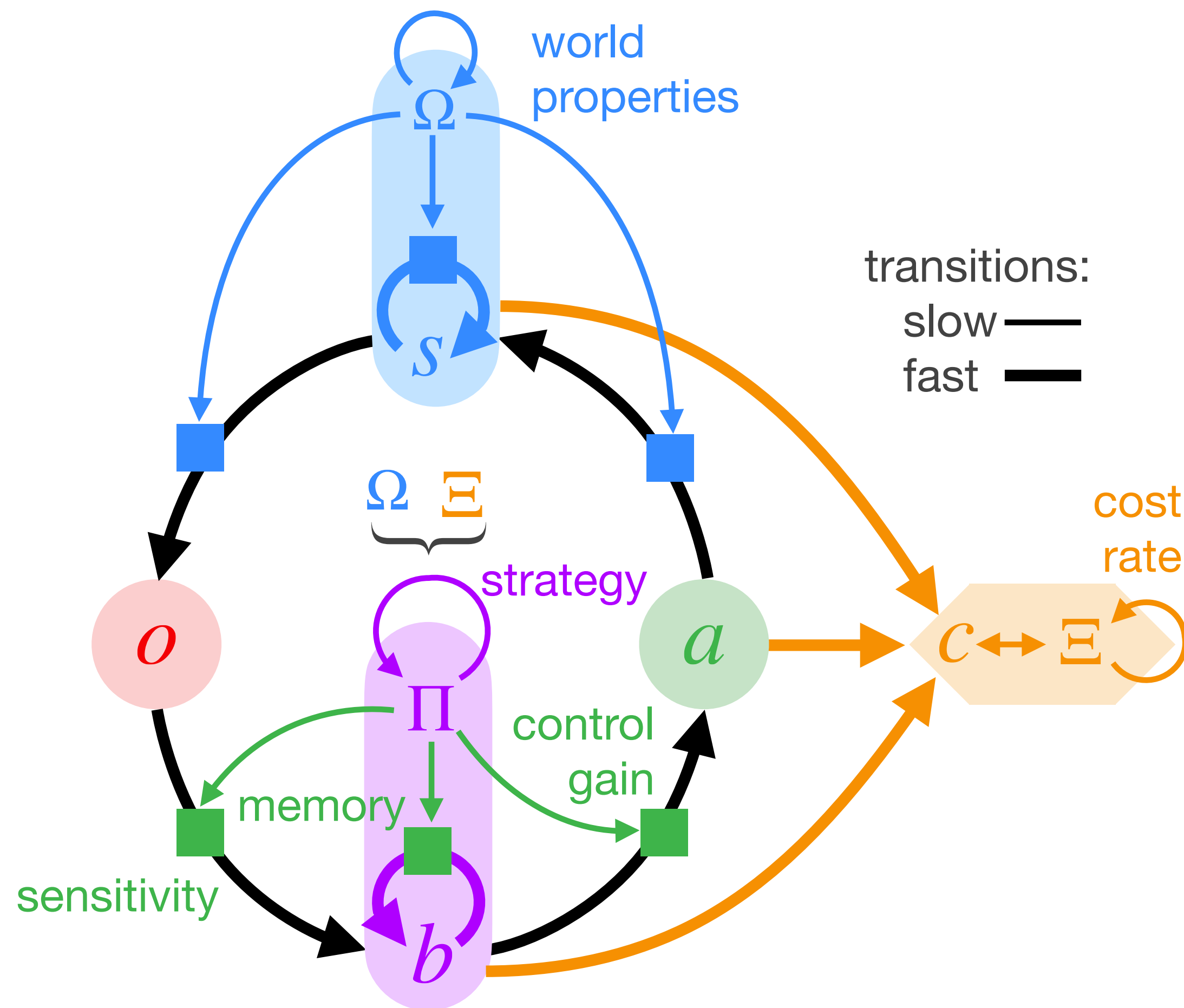
B Frugal POMDP
