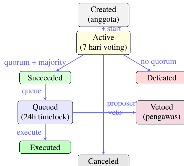
Gambar 3.3. Siklus Hidup Proposal pada LakomiGovern
