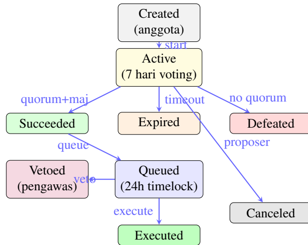
Gambar 3.4. Siklus Hidup Proposal pada LakomiGovern
