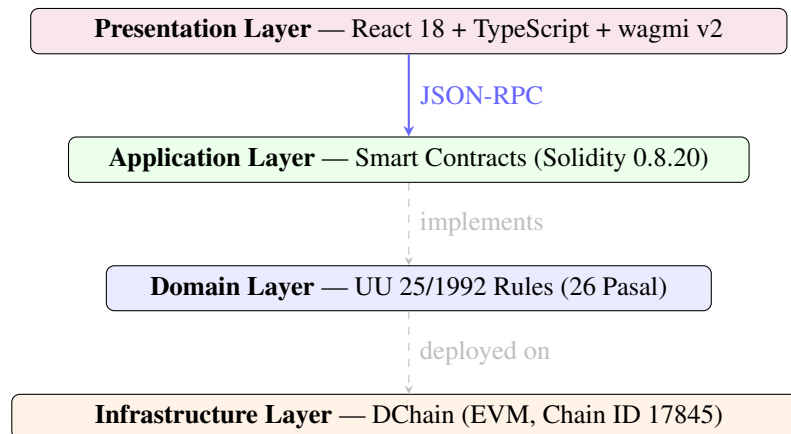
Gambar L.2. Arsitektur Clean Architecture Sistem Lakomi
