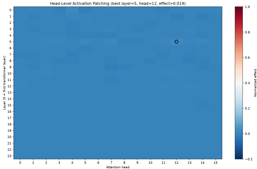
Abbildung 11: Patching auf Ebene einzelner Attention Heads an Position 3 (Token „delicious“).
