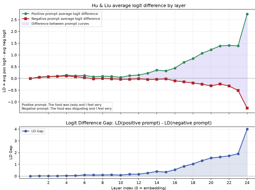
Abbildung 5: Logit-Differenz je Schicht für ein Beispiel-Prompt-Paar, oben die Differenz je Prompt, unten die Lücke zwischen positivem und negativem Prompt.
