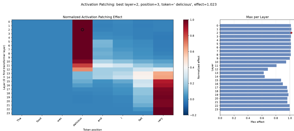
Abbildung 10: Normalisierter Activation-Patching-Effekt über alle Schichten und Token-Positionen.
