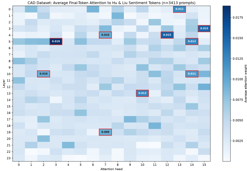
Abbildung 9: Durchschnittliche Aufmerksamkeit je Schicht und Kopf auf sentimenttragende Wörter über den CAD-Datensatz (n=3413 Prompts).
