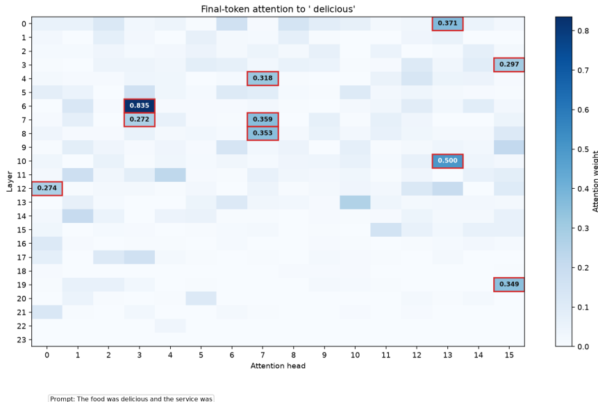
Abbildung 8: Aufmerksamkeit der Köpfe auf das sentimenttragende Token „delicious“ an einem Beispielsatz.
