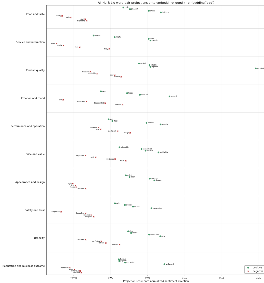
Abbildung 5: Projektion der Sentiment-Wörter auf die Richtung „good“ minus „bad“, getrennt nach thematischen Feldern.
