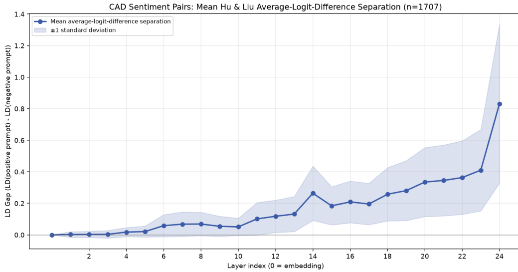
Abbildung 9: Über 1.707 CAD-Paare gemittelte Logit-Differenz je Schicht (Mittelwert \pm 1 Standardabweichung).
