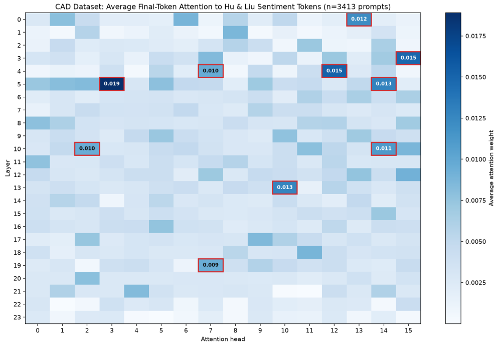
Abbildung 11: Durchschnittliche Aufmerksamkeit je Schicht und Kopf auf sentimenttragende Wörter über den CAD-Datensatz (n=3413 Prompts).
