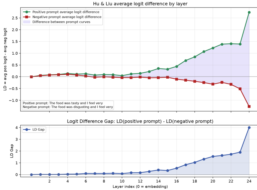
Abbildung 7: Logit-Differenz je Schicht für ein Beispiel-Prompt-Paar, oben die Differenz je Prompt, unten die Lücke zwischen positivem und negativem Prompt.
