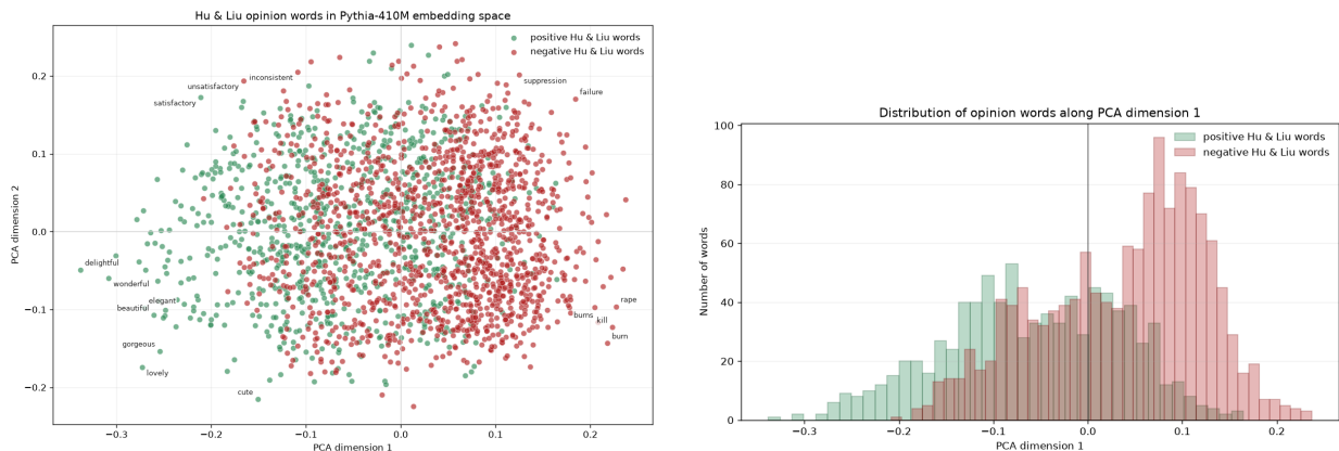
Abbildung 3: Hu-&-Liu-Wörter im Raum der ersten beiden Hauptkomponenten (links) und ihre Verteilung entlang der ersten Hauptkomponente (rechts).
