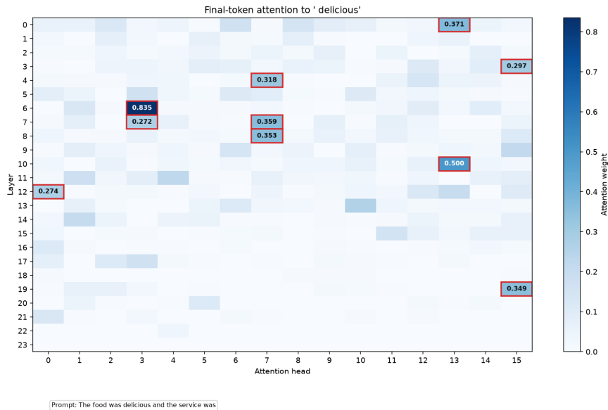
Abbildung 10: Aufmerksamkeit der Köpfe auf das sentimenttragende Token „delicious“ an einem Beispielsatz.
