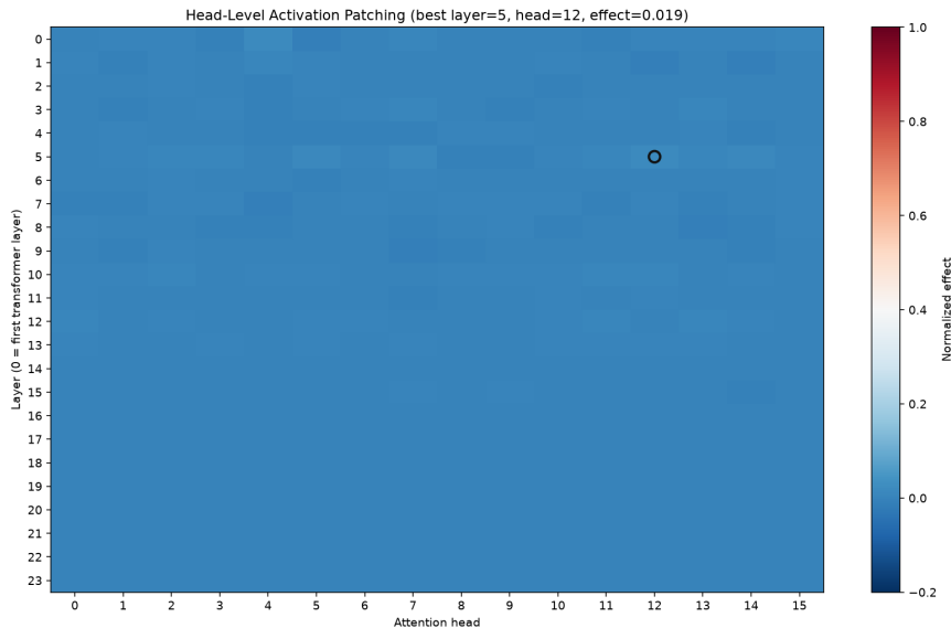
Abbildung 13: Patching auf Ebene einzelner Attention Heads an Position 3 (Token „delicious“).
