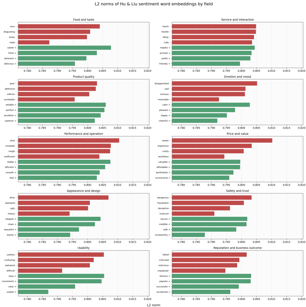
Abbildung 4: L2-Normen der Sentiment-Embeddings getrennt nach thematischen Feldern.
