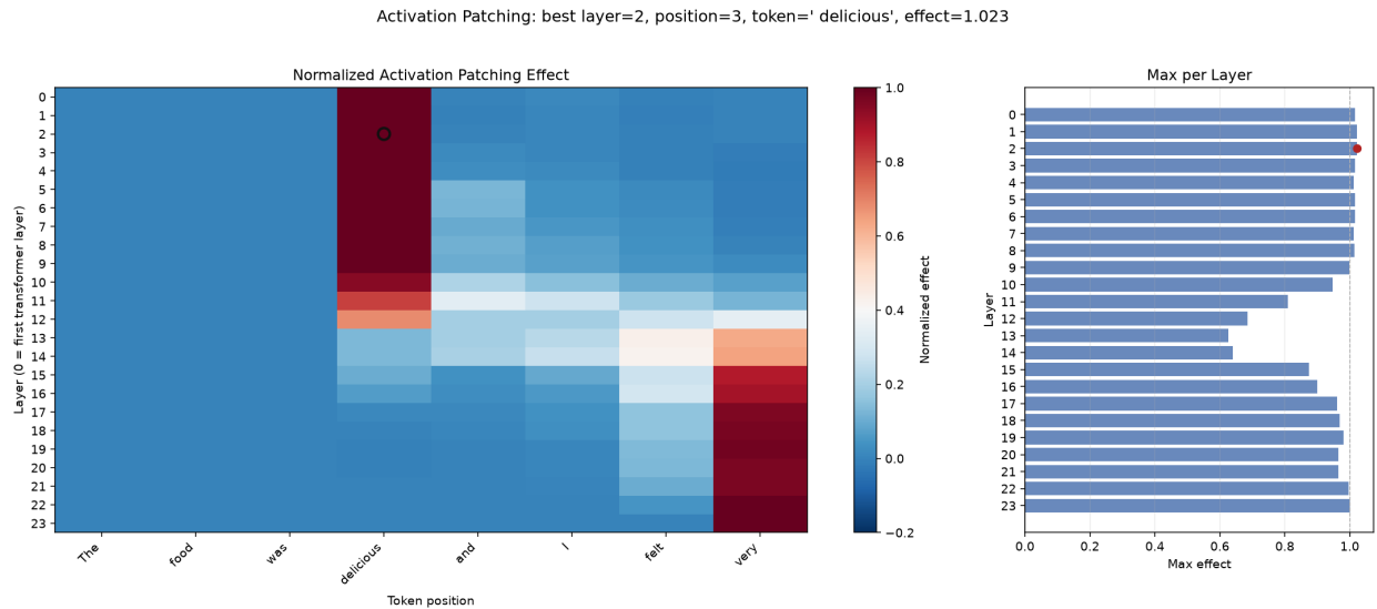
Abbildung 12: Normalisierter Activation-Patching-Effekt über alle Schichten und Token-Positionen.
