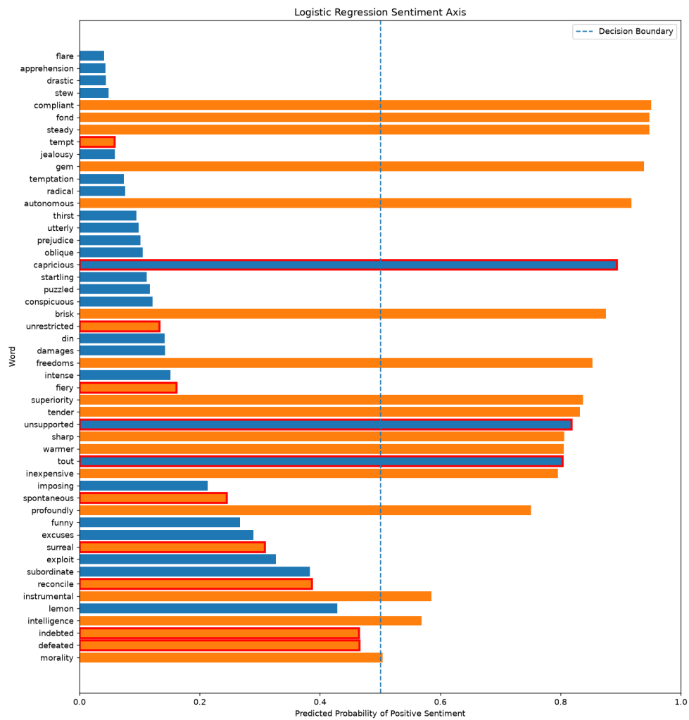
Abbildung 6: Durch die lineare Probe gelernte Sentiment-Achse; falsch klassifizierte Wörter sind rot markiert.
