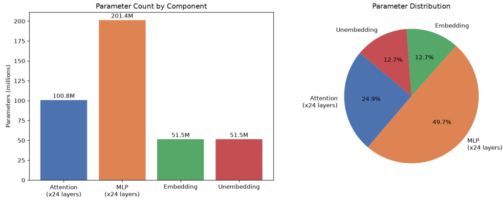
Abbildung 1: Parameterverteilung von Pythia-410M auf Embedding, Attention, MLP und Unembedding.
