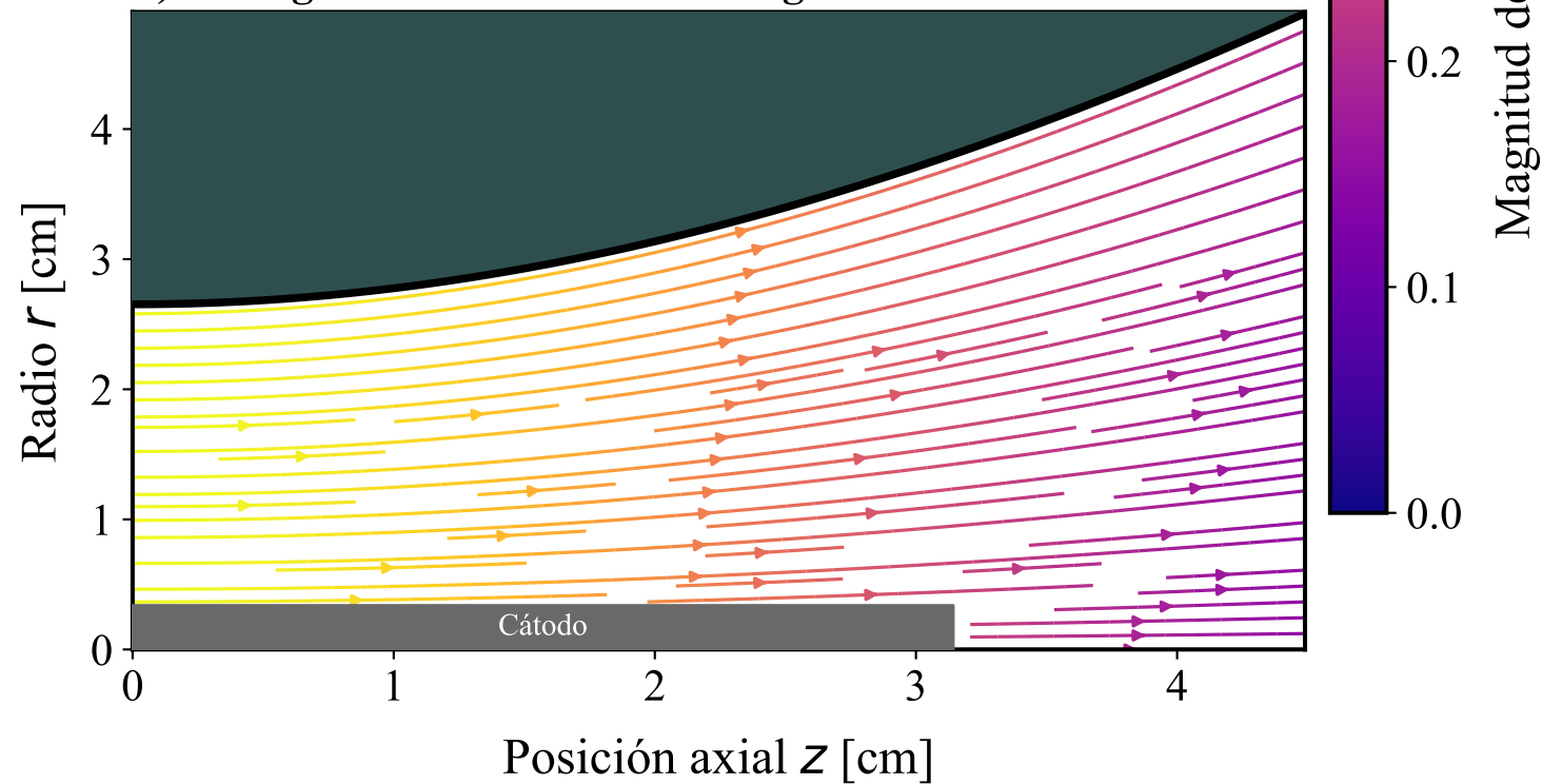
b) Configuración de Tobera Divergente
