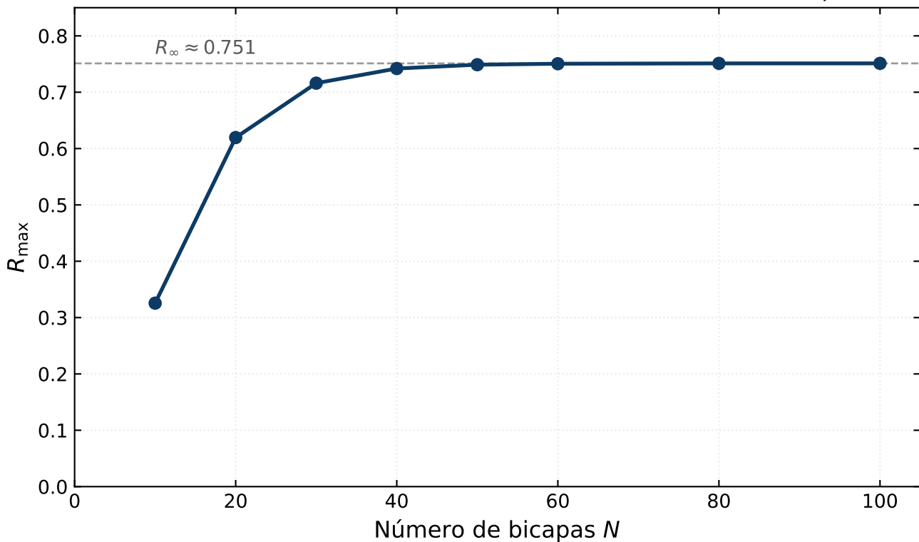
Saturación de la reflectancia máxima con el número de bicapas
