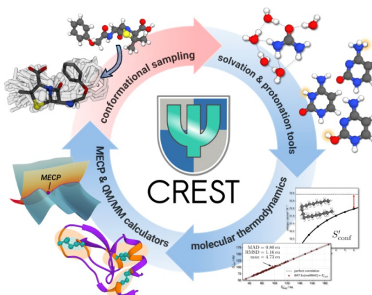
図 2 使用した CREST 概要
