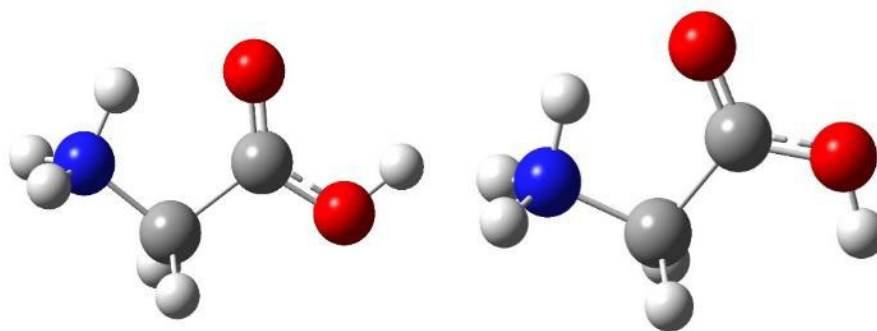
図 1 Chemcraft で可視化されたグリシンの構造の一例
