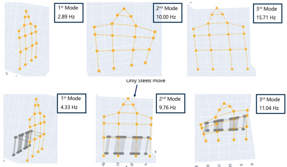
図 3 固有値解析の結果（上段：Facade のみ、下段：Facade+鉄筋）
