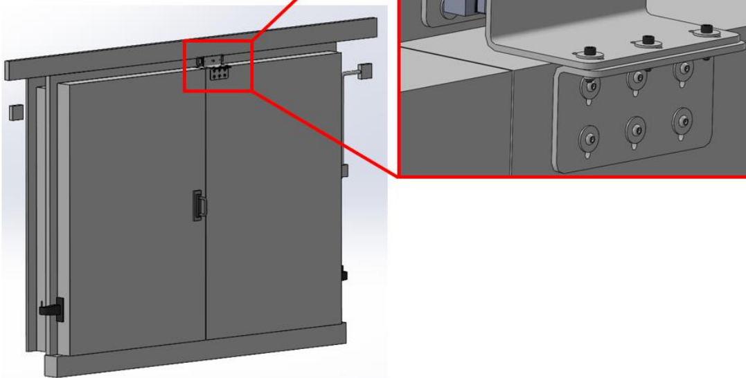
車庫扉の開閉マグネットの配置検討
