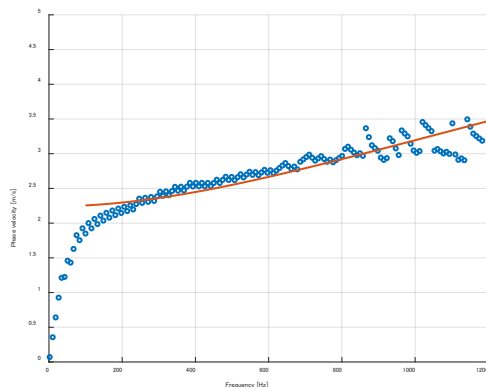
Kelvin-Voigt モデル
