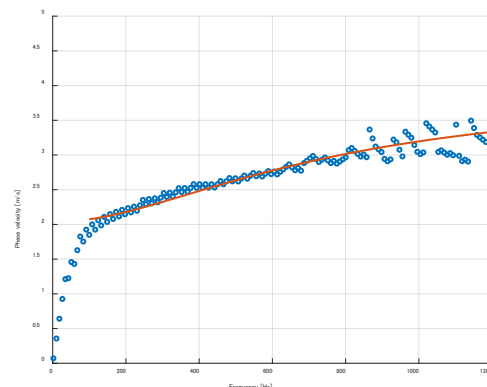
Zener モデル
