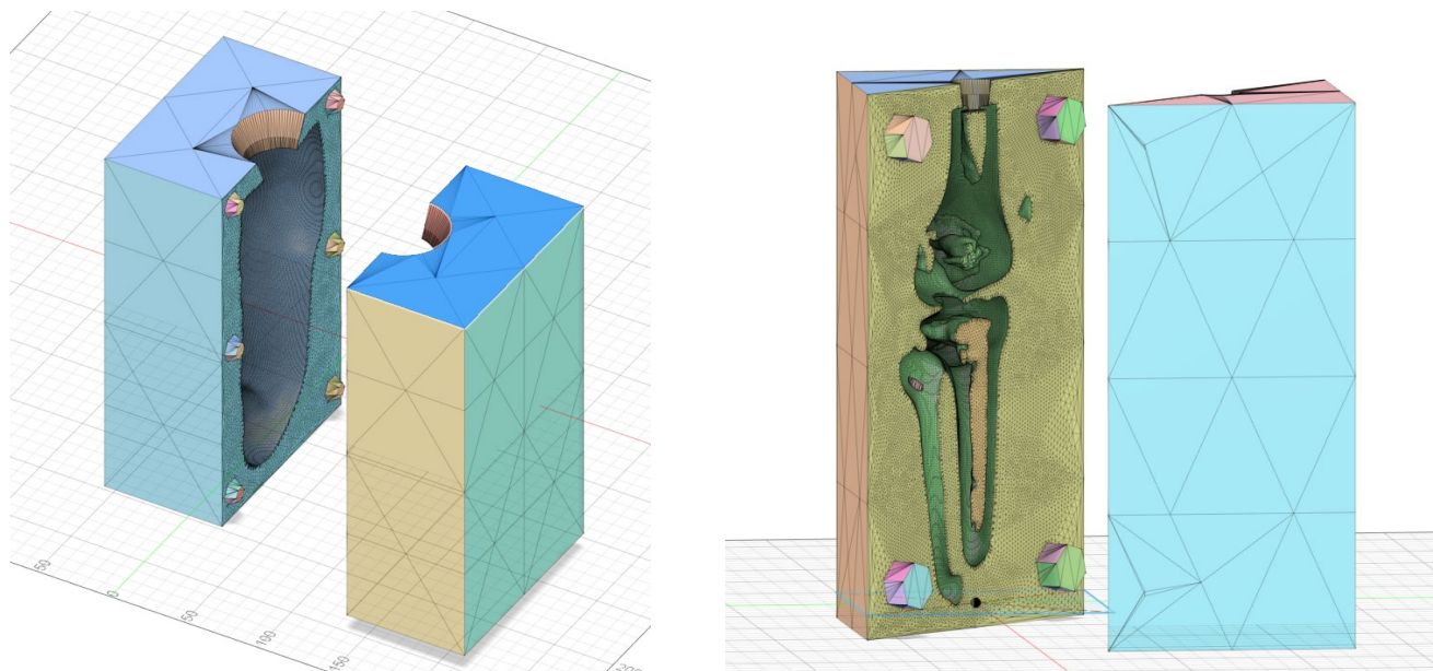
図 CADで作製した型（左:皮膚型 右:骨型）
