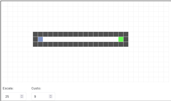
Figure 5: Mapa em que a DFS retorna a solução ótima.
