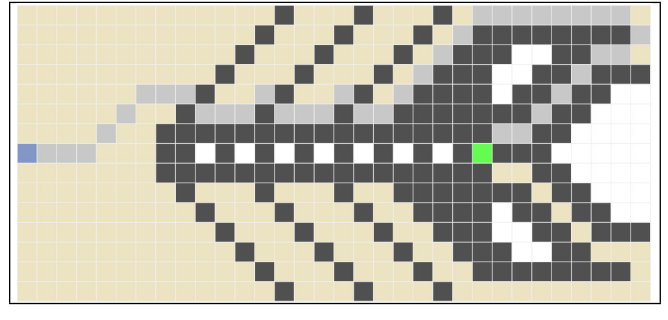
Figure 15: Solução de ambas as buscas.
