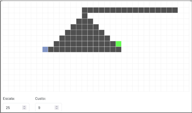
Figure 7: Mapa em que o Greedy é ótimo.
