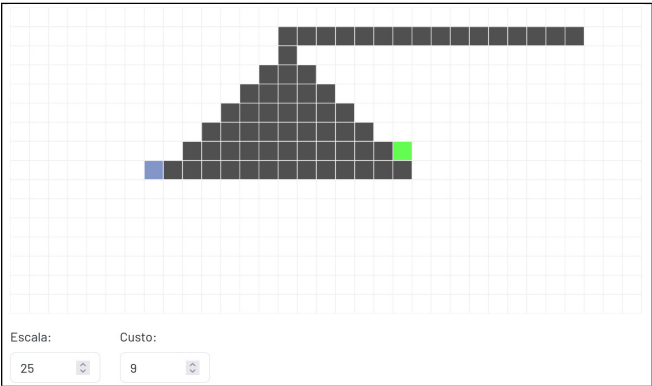
Figure 9: Mapa em que o Greedy não é ótimo.
