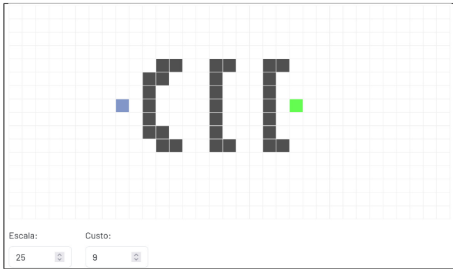
Figure 11: Mapa em que o A^* é melhor que UCS.
