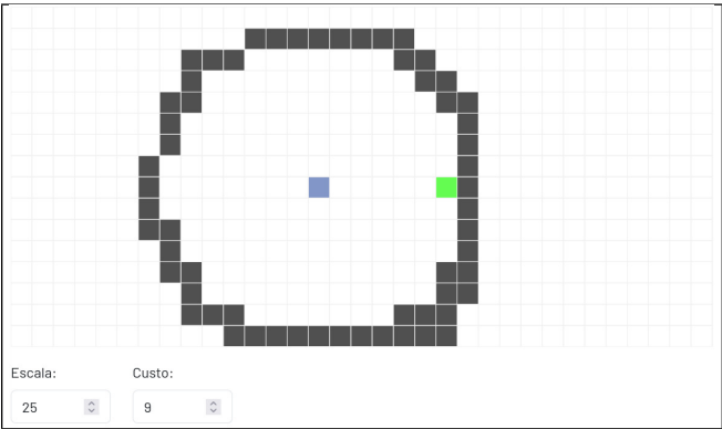
Figure 3: Mapa em que a BFS é equivalente à UCS.
