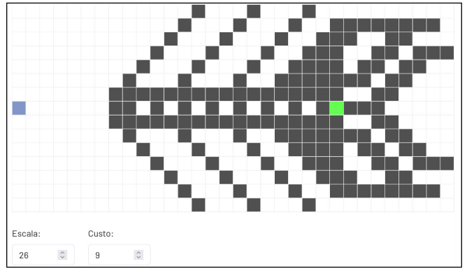
Figure 14: Mapa em que o A^* é equivalente a UCS.
