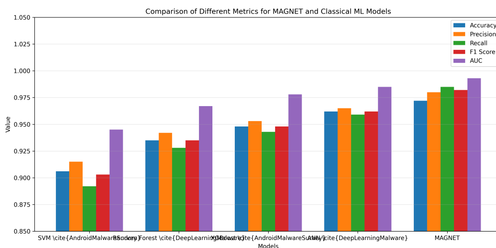
شکل ۹-۵. مقایسه Score F1 و AUC مدل MAGNET با سایر مدل‌ها.
