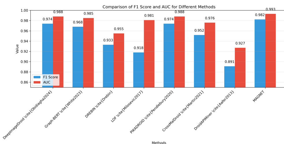
شکل ۵-۸. مقایسه Score F1 و AUC روش‌های مختلف.
