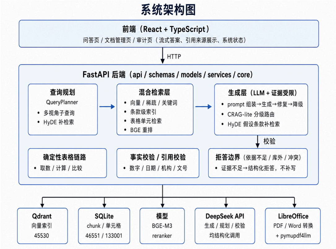
ReguMate 系统架构图
