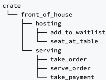
示例 7-2: 示例 7-1 中代码对应的模块树
