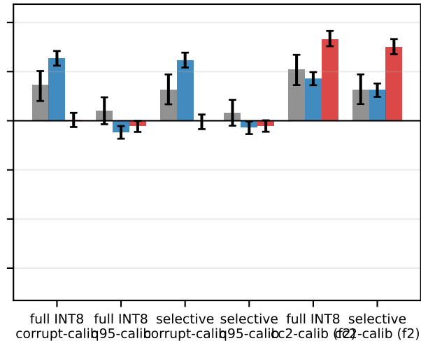
VOC
