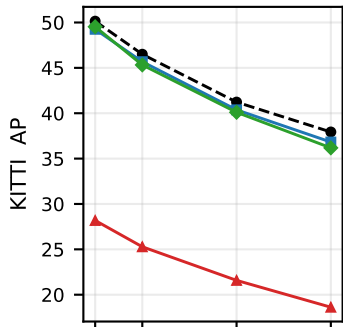
Fog
