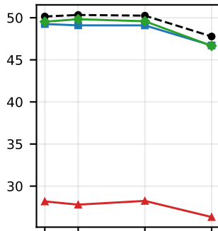
JPEG
