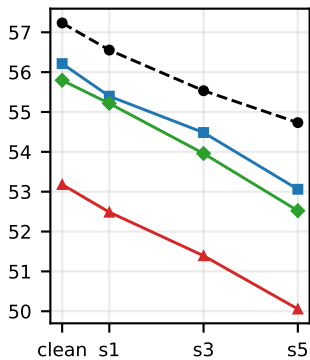
VOC AP
