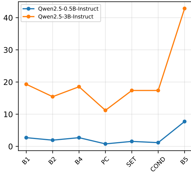
musique
