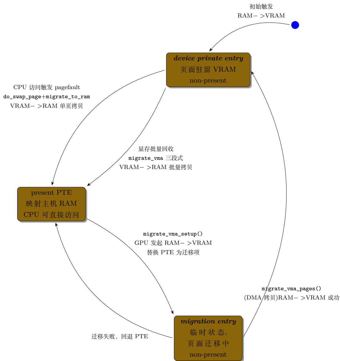
图 10-6: HMM 设备私有页 PTE 状态转换图
