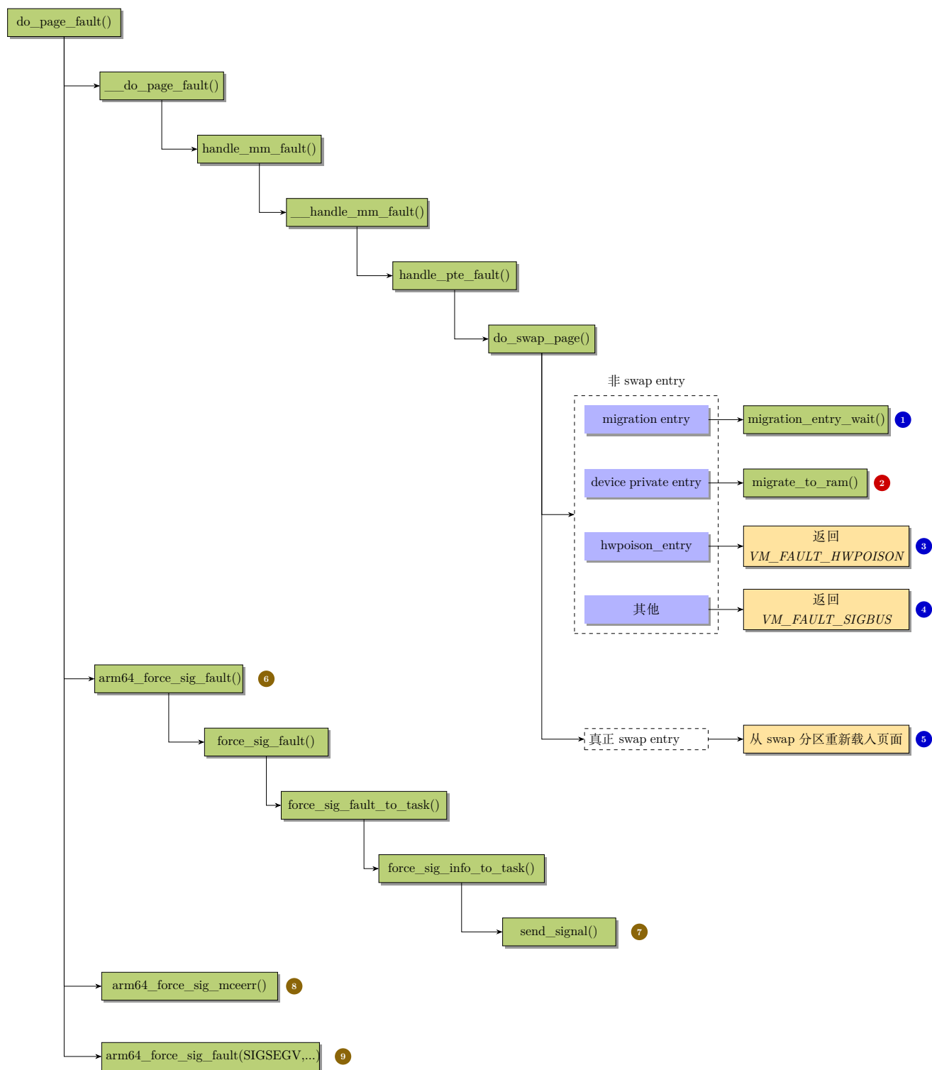
图 10-1: do_page_fault() 的调用栈
