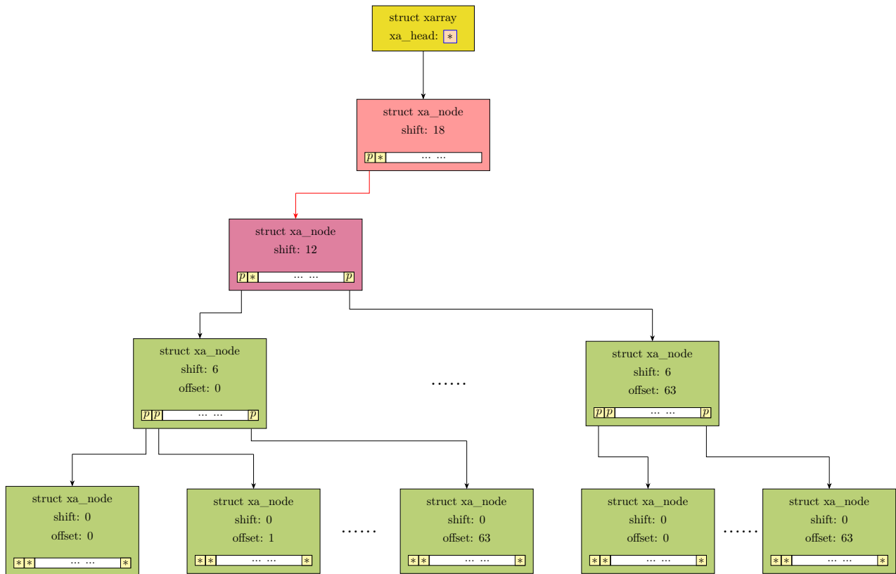
图 14-5: xarray 继续扩容，挂接到 shift=18 的新顶层父节点
