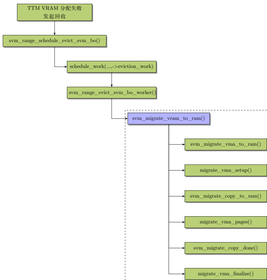
图 10-5: 内存压力触发的 VRAM → RAM 批量迁移的执行流
