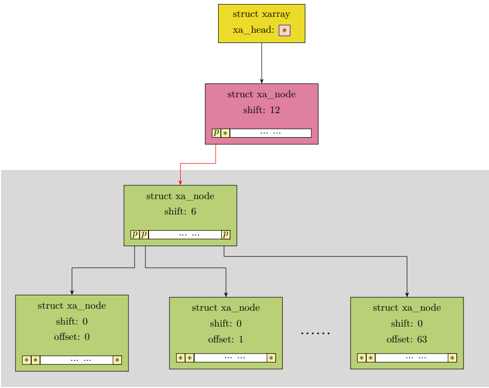
图 14-4: xarray 扩容，挂接到 shift=12 的新顶层父节点
