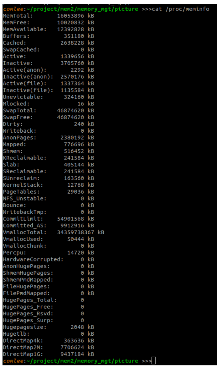
图 12-2: /proc/meminfo 节点的输出信息
