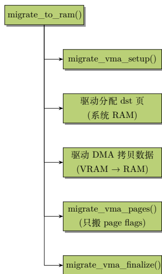
图 10-2: migrate_to_ram() 的部分执行逻辑
