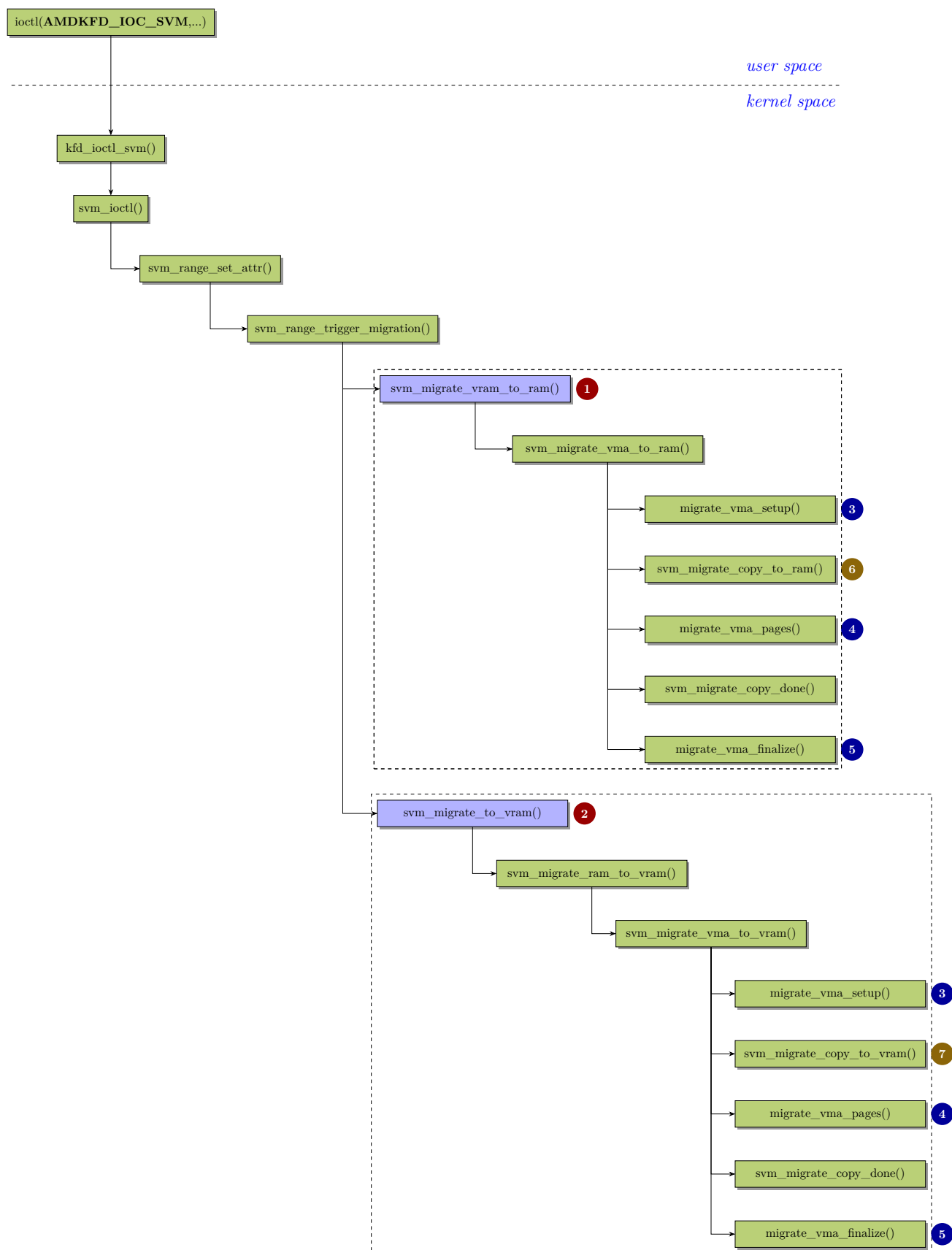
图 10-4: ioctl() 触发的批量迁移的执行流
