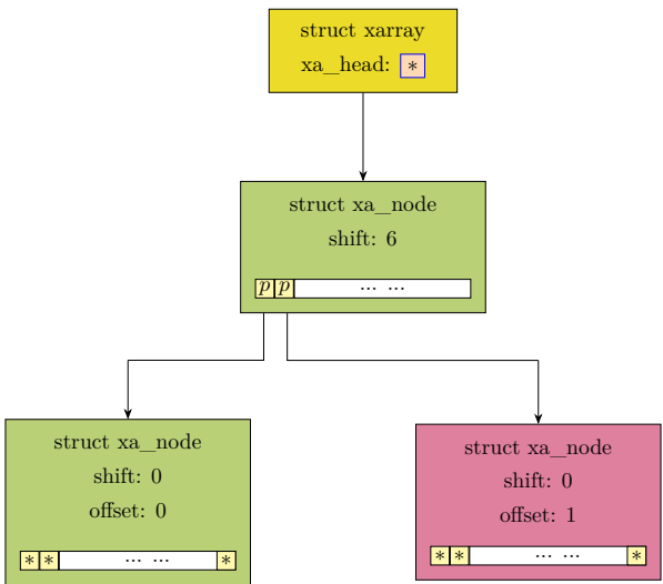
图 13-2: 新建的第二个叶节点填充到父节点 (shift=6) 的 slot[1] 槽
