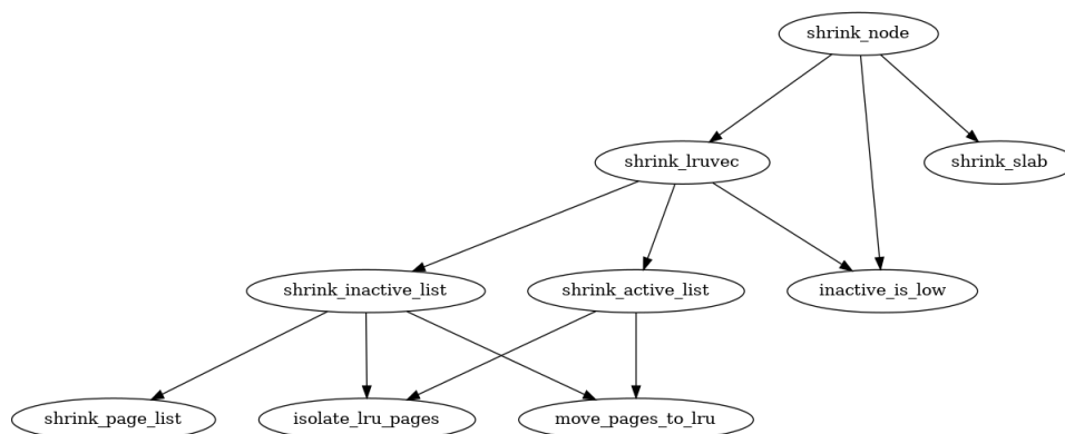
图 5-3: 调用图: shrink_node()
