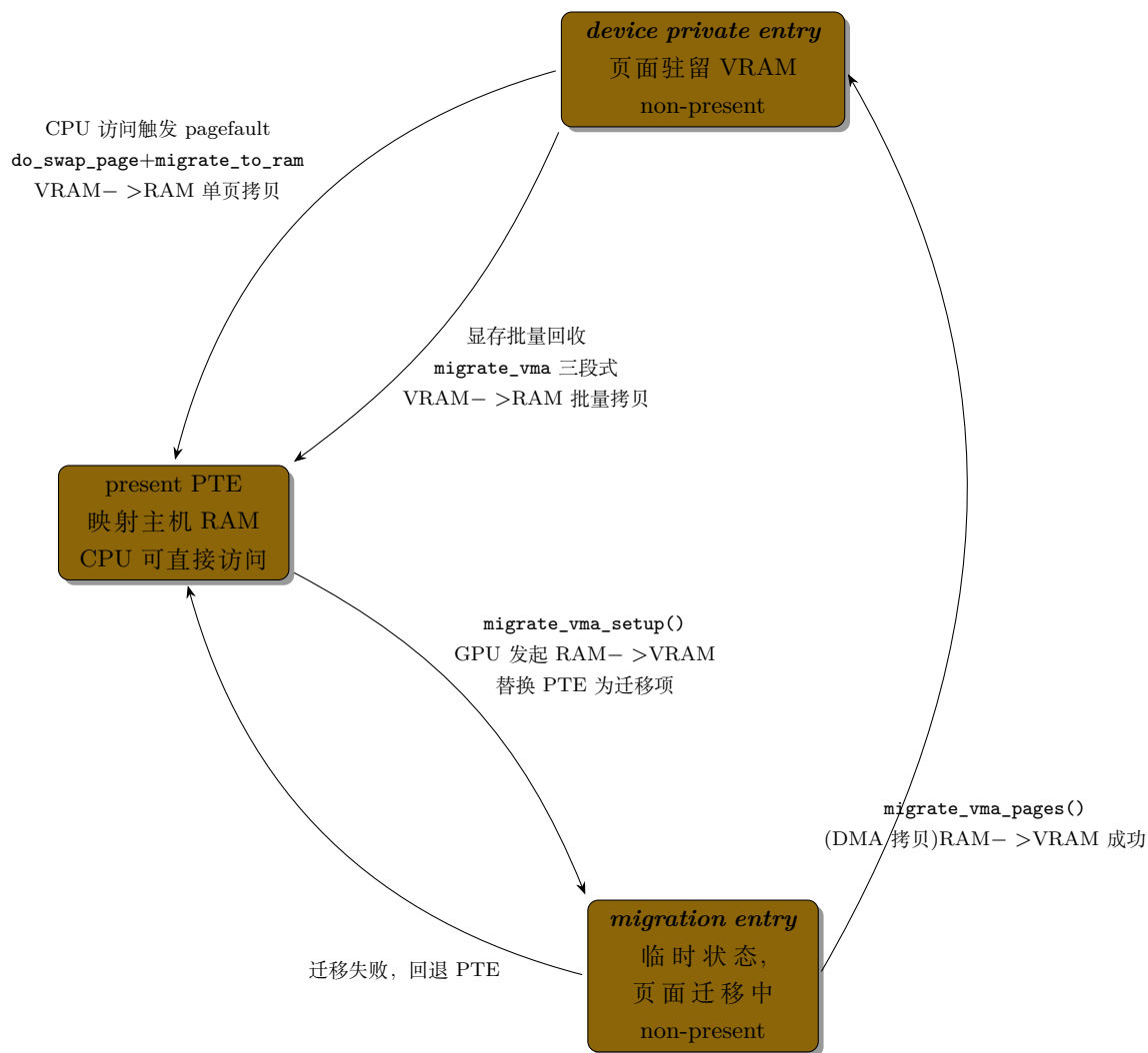
图 10-4: HMM 设备私有页 PTE 状态转换图
