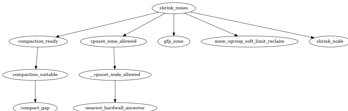
图 5-2: 调用图：shrink_zones()
