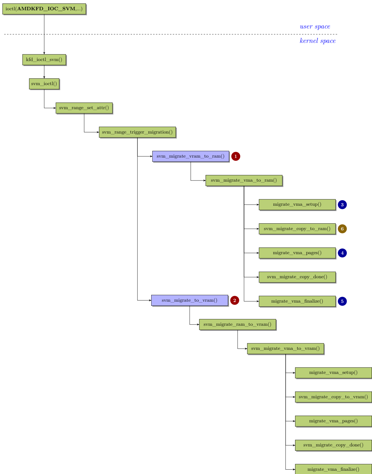
图 10-3: ioctl() 触发的批量迁移的执行流
