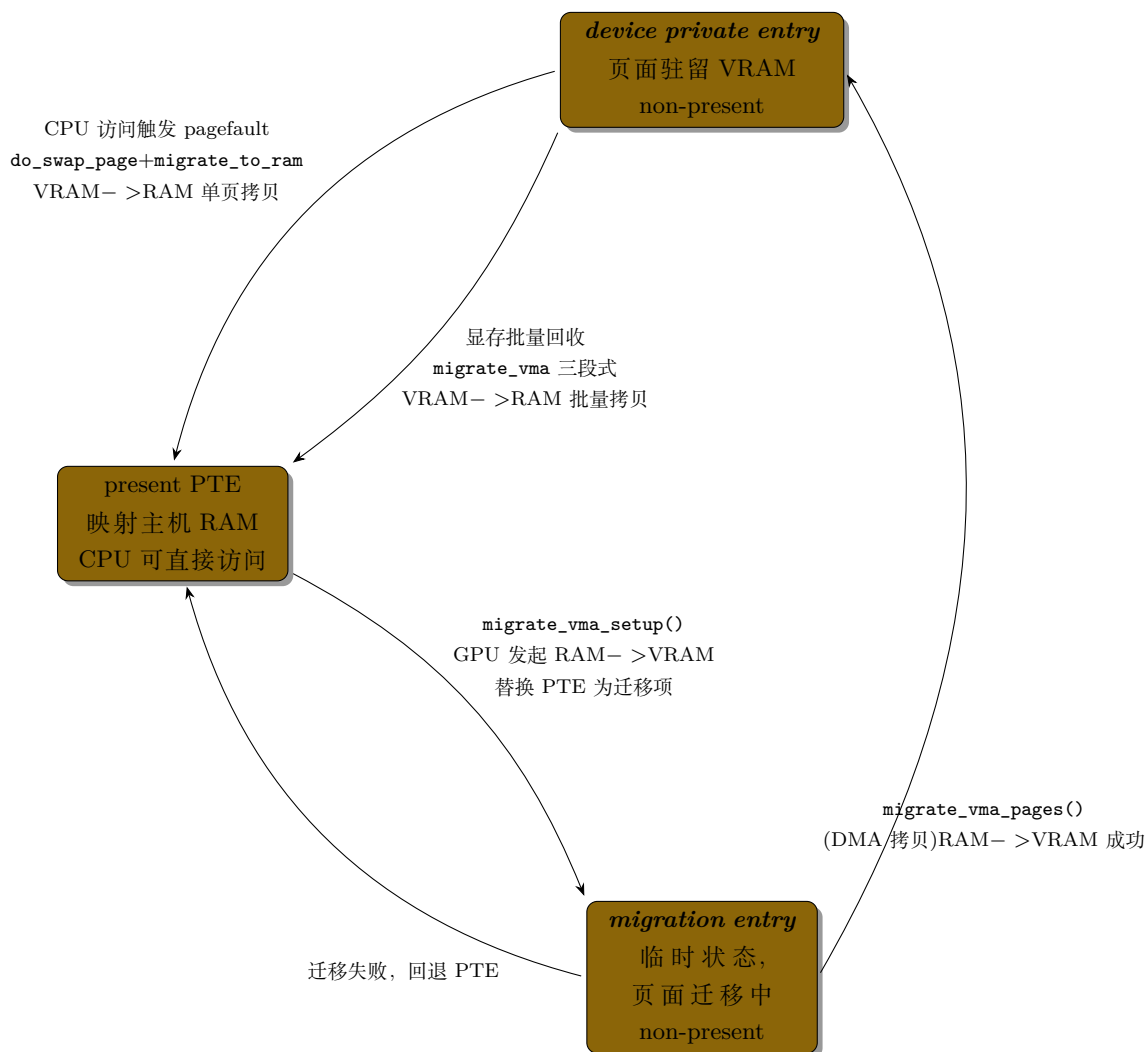
图 10-5: HMM 设备私有页 PTE 状态转换图
