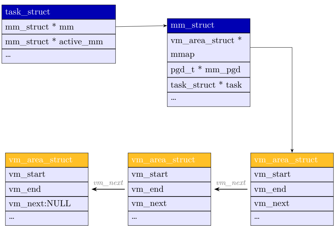
图 9-1: task_struct 、 mm_struct 、 vm_area_struct 数据结构关系
