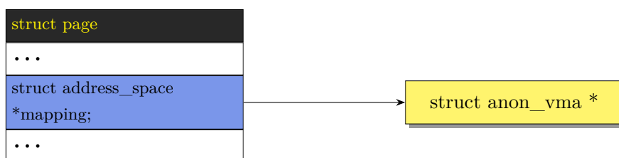
图 9-2: pagecache 和匿名页的 mapping 指向不同对象
