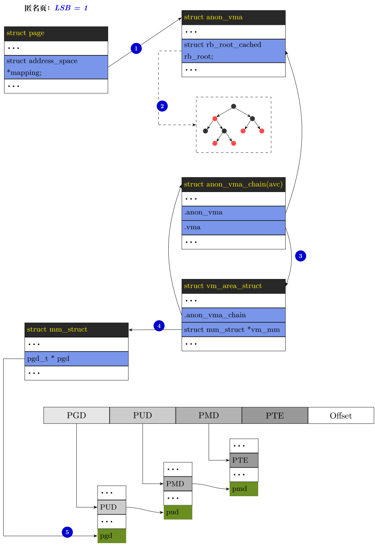
图 9-3: 反向映射: 匿名页查找 PTE 的流程
