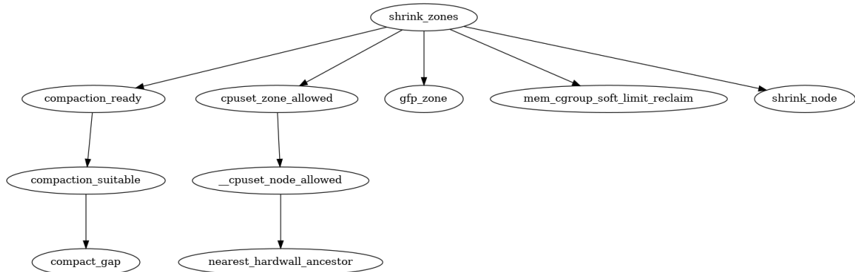
图 5-2: 调用图：shrink_zones()
