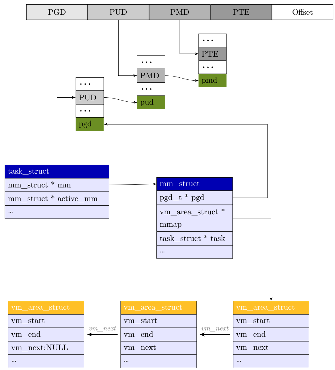
图 9-1: 正向映射: 从 task_struct 查找 mm_struct(mm), 再通过 mm->pgd 和虚拟地址检索页表, 定位到 PTE
