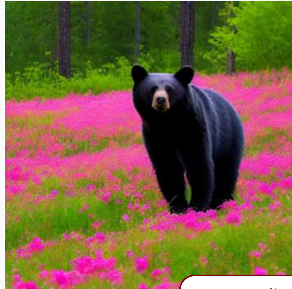
w/o Prompt2Prompt
