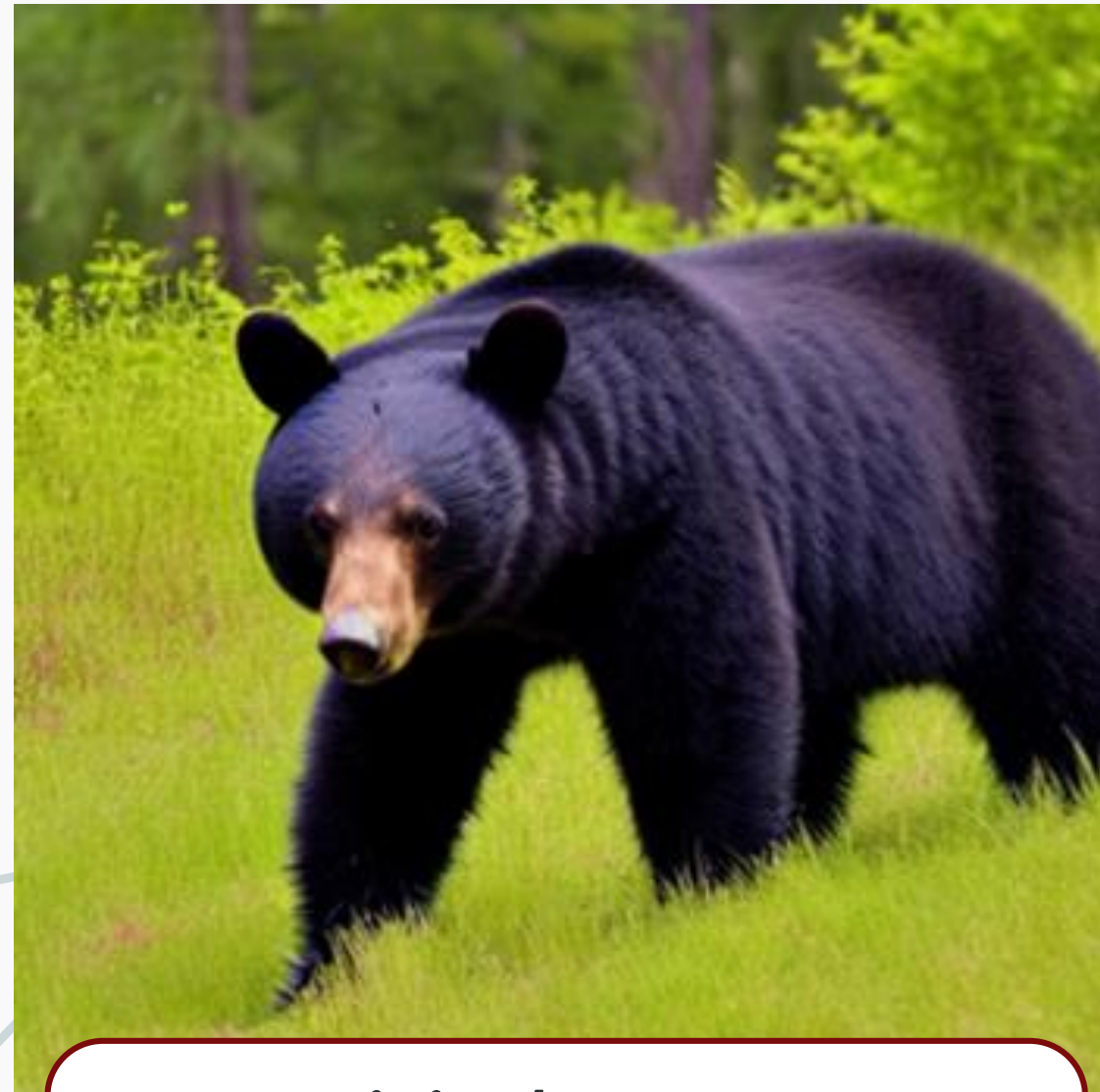
Stable Diffusion
