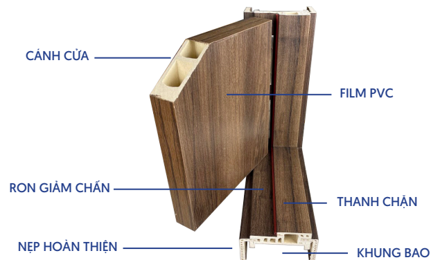
GÓC CỬA MIVIDOOR
