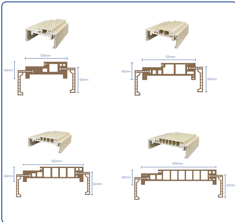
MẶT CẮT KHUNG BAO
