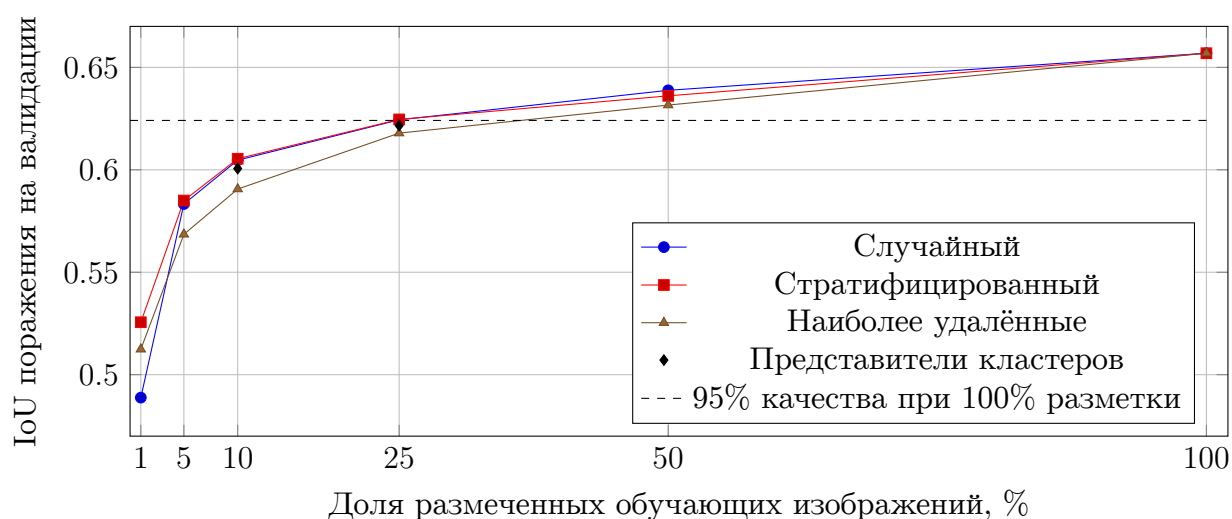
Рис. 5.2 – Кривые эффективности разметки при фиксированном числе шагов. Пунктиром показан уровень 0.6241 — 95% от IoU, полученного при обучении на всей доступной разметке.
