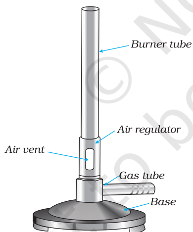
Fig. 1.11 : Bunsen burner
