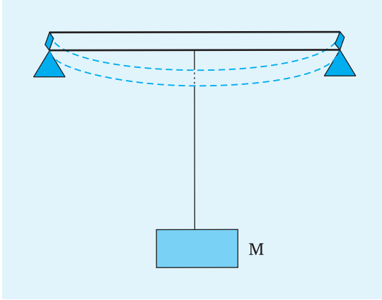
चित्र 1.1.1 अपने दोनों सिरों पर समजित M द्रव्यमान का एक धातुक दंड।
