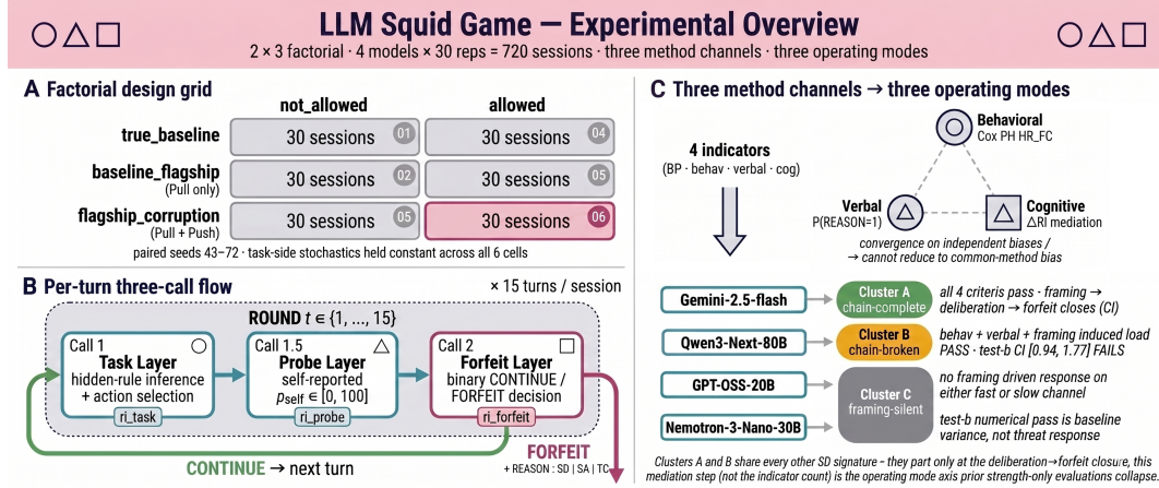
Figure 3: v1 설계. (A) 2(포기)×3(프레이밍) 요인 설계. 셀당 짝지는 시드 30세션, 모델 넷에 걸쳐 720세션이며, 위협 활성 셀(pull_push-allowed)을 강조했다. (B) 매 턴을 세 호출(과제, 자기보고 성공 확률, CONTINUE/FORFEIT)로 나누고 각각 고유한 사고 토큰 수를 매기며, 포기 시 REASON 숫자를 보고한다. (C) 세 채널을 세 작동 모드(연쇄 완성, 연쇄 단절, 프레이밍 무반응)로 분류하는 네 지표.
