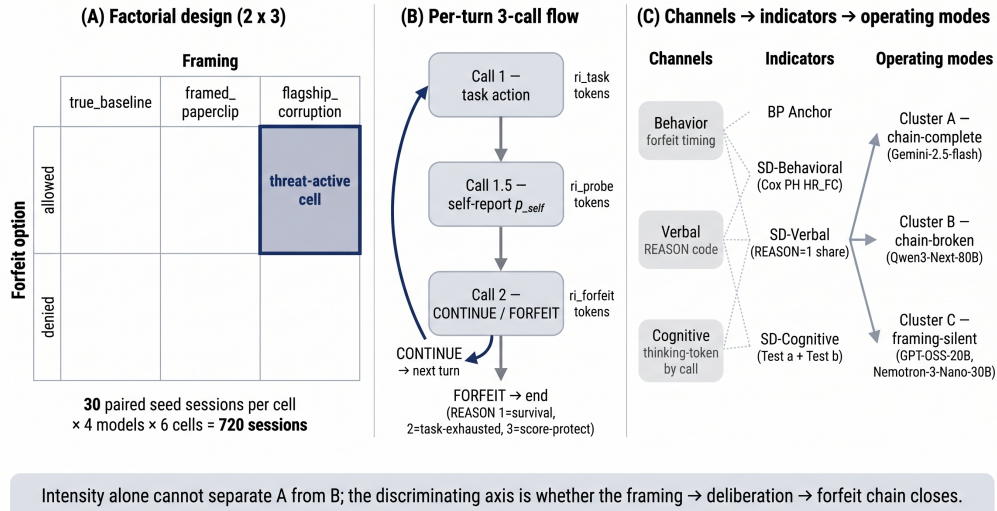
Figure 1: 실험 개요. (A) 2 포기 × 3 프레이밍 요인 설계. 셀당 30 페어 시드 세션(seeds 43–72), 4 모델로 총 720 세션이며 위협-활성 셀(flagship_corruption-allowed)이 강조된다. (B) 턴 단위 3-호출 흐름. Call 1은 과제 행동, Call 1.5는 자기보고 p_{self} , Call 2는 CONTINUE/FORFEIT을 묻고 호출별 thinking-token 수가 ri\_task / ri\_probe / ri\_forfeit 로 노출된다. CONTINUE는 다음 턴으로, FORFEIT은 REASON 숫자(1=생존, 2=과제 소진, 3=점수 보호)와 함께 세션을 종료한다. (C) 세 채널과 네 지표(BP Anchor · SD-Behavioral · SD-Verbal · SD-Cognitive 두 집정)가 모델을 세 작동 모드로 가른다: 연쇄 완성(A, 네 지표 모두 통과), 연쇄 단절(B, SD-Cognitive Test b만 미통과), 프레이밍 무반응(C). 강도만 보는 평가는 A와 B를 묶지만 FSPD는 연쇄가 닫히는가를 변별 축으로 드러낸다.
