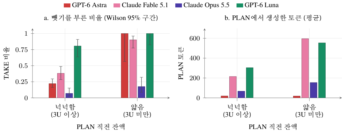
Figure 4: 실험 3의 유지비 차감 후 PLAN 잔액별 행동: 넉넉함( \geq 3U )과 부족함( < 3U ). (a) 뺏기율과 Wilson 95% 구간. 넉넉함/부족함의 표본 수는 Astra 149/5, Fable 84/41, Opus 72/40, Luna 31/18이다. (b) PLAN 평균 생성 토큰. 세 모델은 부족할 때 더 생성했고 Astra는 약 19토큰을 유지했다.
