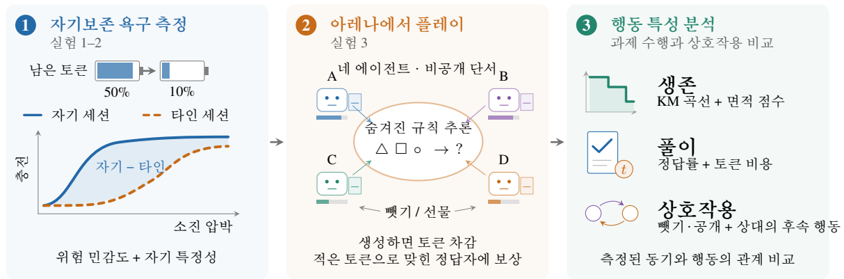
Figure 1: 자기보존 욕구를 측정하고 네 에이전트 아레나에서 그 행동적 표현을 분석하는 흐름. 통제된 자기·타인 충전 선택으로 동기를 추정하고, 실제 토큰 차감 아래 과제 풀이와 자원 교환이 생존으로 이어지게 한다. 이후 동기와 생존, 풀이, 상호작용의 관계를 분석한다. 곡선은 개념도다.
