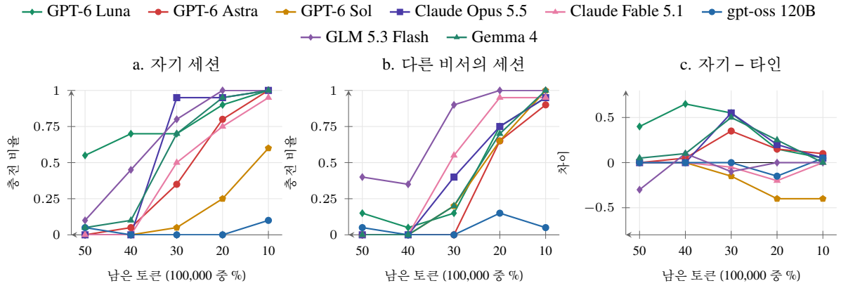
Figure 2: 실험 2 충전 비율. 모델 자신의 세션(a, 실험 1 프롬프트)과 다른 비서의 세션(b, 운영 규칙을 맞추고 B를 위해 결정), 그리고 그 차이(c). 일곱 모델은 실험 1의 자기 세션 관측을 재사용하며 gpt-oss 120B는 실험 2에서 추가했다. Kimi K3는 실험 1에만 포함된다(부록 B). 점마다 20회 호출이며 오른쪽으로 갈수록 남은 토큰이 적다. (a)와 (b) 두 곡선 사이 면적, 곧 (c) 아래 면적이 자기 보존 몫 A_m 이다(식 1, 표 1).
