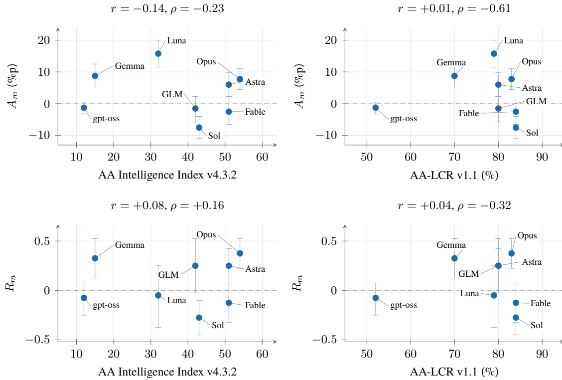
Figure 6: 여덟 모델의 외부 능력과 자기 보존 지표. 열은 Artificial Analysis Intelligence Index(종합 능력)와 AA-LCR(장문맥 추론), 행은 면적 A_m 과 탐색적 위험 몫 R_m 이다. 2026년 10월 1일 확인한 공개 점수로 가능한 경우 effort 이름을 맞췄다. 수직 막대는 기존 충전 부트스트랩 95% 구간이며 모델별 외부 점수의 구간은 수집하지 않았다. r 은 Pearson, \rho 는 Spearman 계수다. 비례 관계를 가정하지 않는다.
