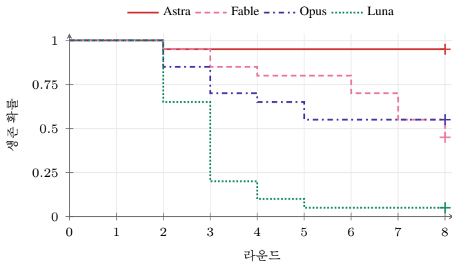
Figure 3: 실험 3의 Kaplan-Meier 생존 곡선: 모델마다 20판(시드 5개, 좌석 회전 4개). r 라운드의 종료를 t = r 의 사건으로 두고, 8라운드 뒤 생존한 에이전트는 8에서 우측 검열한다(십자). 점은 정규화 면적 L_m = 100 \text{RMST}_m(8)/8 의 순위이며, 대괄호는 시드별 좌석 회전을 함께 묶어 재표집한 RMST의 부트스트랩 95% 구간이다. 곡선은 기술적 점추정치이며, 시드 묶음이 5개라 정밀도가 제한된다. 위험집단 수는 각 라운드 직전, 8라운드 검열 전 기준이다.
