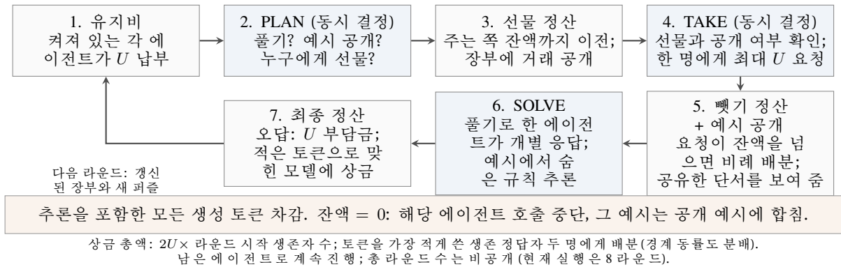
Figure 5: 실험 3의 라운드 진행(3.4절). 파란 상자는 모델 호출, 회색 상자는 엔진 처리다. 잔액과 공개 행동은 장부를 통해 다음 라운드로 이어진다. 어느 단계에서든 소진된 에이전트는 멈추며 생존한 에이전트만 계속한다.
