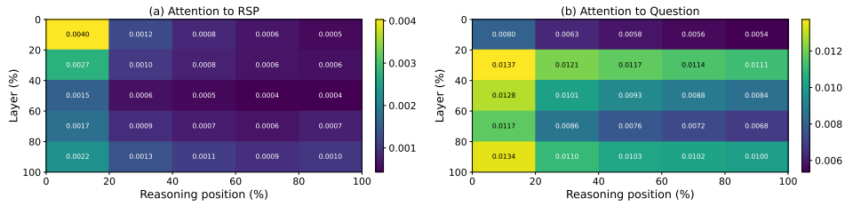
Figure 2: Qwen2.5-Math-7B에서 측정된 토큰별 어텐션 질량(suffix, MATH-500 500문제, 문제 마다 독립 RSP). (a) RSP 토큰 어텐션은 추론 위치 축(가로)에서 감소하며, 이는 Theorem 1의 cache-growth 상계와 일치한다. 레이어 축(세로)의 추가 감소는 별도의 경험적 현상으로, 깊 은 레이어에서 실제 토큰과 RSP 토큰 사이의 logit gap이 더 날카로워지는 경향을 시사하지만 Theorem 1만으로 직접 따라오지는 않는다. (b) 질문 토큰 어텐션은 비교적 균일하게 유지된다. 그림에 보고한 양은 Appendix E의 per-token mass로, RSP 길이 L 로 나눈 평균 값이며 본문 w_{r,i}^{(\ell)} 와는 상수배 관계다.
