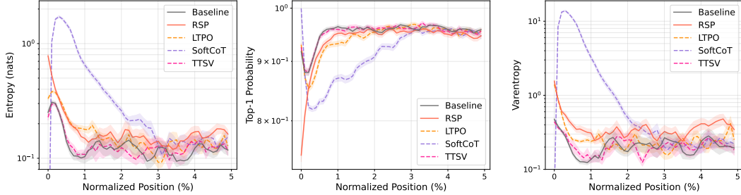
Figure 3: 생성 초반 5% 구간의 평균 entropy, top-1 probability, varentropy (Qwen2.5-Math-1.5B-Instruct, MATH-500). 음영은 \pm 1 SEM이다. 실선은 RSP 변형과 baseline, 점선은 기존 soft prompt 방법(LTPO, SoftCoT, TTSV)이다.
