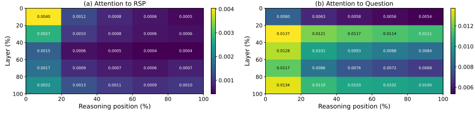
Figure 2: Qwen2.5-Math-7B에서 측정한 토큰별 어텐션 질량(suffix, MATH-500 500문제, 문제마다 독립 RSP). (a) RSP 토큰 어텐션은 추론 위치 축(가로)에서 감소하며, 이는 Theorem 1의 cache-growth 상계와 일치한다. 레이어 축(세로)의 추가 감소는 별도의 경험적 현상으로, 깊은 레이어에서 실제 토큰과 RSP 토큰 사이의 logit gap이 더 날카로워지는 경향을 시사하지만 Theorem 1만으로 직접 따라오지는 않는다. (b) 질문 토큰 어텐션은 비교적 균일하게 유지된다. 그림에 보고한 양은 Appendix E의 per-token mass로, RSP 길이 L 로 나눈 평균 값이며 본문 w_{r,i}^{(\ell)} 와는 상수배 관계다.
