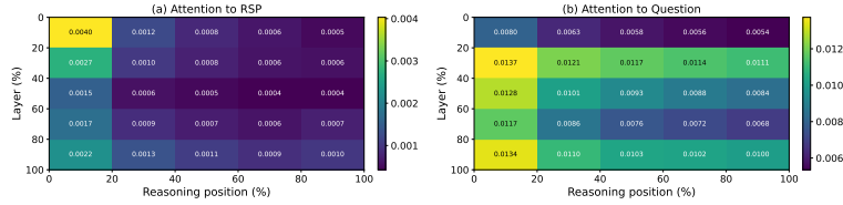
Figure 2: Qwen2.5-Math-7B에서 측정한 토큰별 어텐션 질량(suffix, MATH-500 500문제, 문제 마다 독립 RSP). (a) RSP 토큰 어텐션은 추론 위치 축(가로)에서 감소하며, 이는 Theorem 1의 cache-growth 상계와 일치한다. 레이어 축(세로)의 추가 감소는 별도의 경험적 현상으로, 깊 은 레이어에서 실제 토큰과 RSP 토큰 사이의 logit gap이 더 날카로워지는 경향을 시사하지만 Theorem 1만으로 직접 따라오지는 않는다. (b) 질문 토큰 어텐션은 비교적 균일하게 유지된다. 그림에 보고한 양은 Appendix F의 per-token mass로, RSP 길이 L 로 나눈 평균 값이며 본문 w_{r,i}^{(\ell)} 와는 상수배 관계다.
