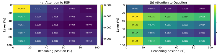
Figure 1: Qwen2.5-Math-7B에서 측정한 토크별 어텐션 질량(suffix, MATH-500 500문제, 문제마다 독립 RSP). (a) RSP 토크 어텐션은 추론 위치 축(가로)에서 감소하며, 이는 Theorem 1의 cache-growth 상계와 일치한다. 레이어 축(세로)의 추가 감소는 별도의 경험적 현상으로, 깊은 레이어에서 실제 토크와 RSP 토크 사이의 logit gap 이 더 날카로워지는 경향을 시사하지만 Theorem 1만으로 직접 따라오지는 않는다. (b) 질문 토크 어텐션은 비교적 균일하게 유지된다. 그림에 보고한 양은 Appendix F의 per-token mass로, RSP 길이 L 로 나눈 평균 값이며 본문 w_{r,i}^{(\ell)} 와는 상수배 관계다.
