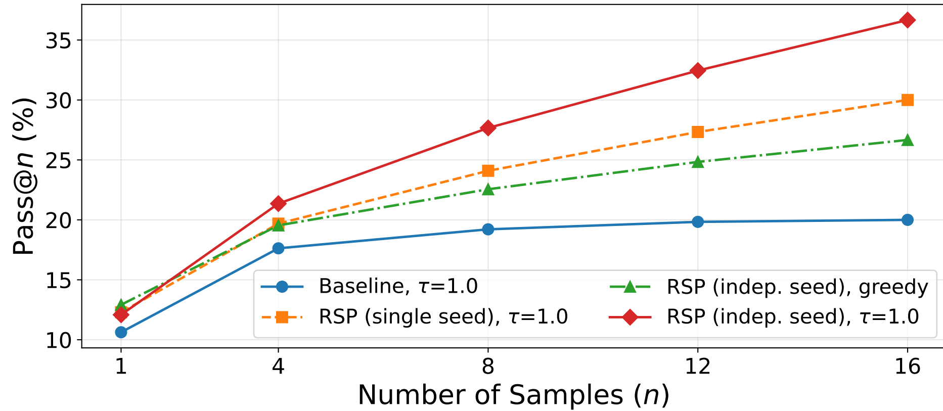
(b) AIME24
