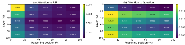
Figure 1: Qwen2.5-Math-7B에서 측정한 토큰별 어텐션 질량(suffix, MATH-500 500문제, 문제마다 독립 RSP). (a) RSP 토큰 어텐션은 추론 위치 축(가로)에서 감소하며, 이는 Theorem 1의 cache-growth 상계와 일치한다. 레이어 축(세로)의 추가 감소는 별도의 경험적 현상으로, 깊은 레이어에서 실제 토큰과 RSP 토큰 사이의 logit gap 이 더 날카로워지는 경향을 시사하지만 Theorem 1만으로 직접 따라오지는 않는다. (b) 질문 토큰 어텐션은 비교적 균일하게 유지된다. 그림에 보고한 양은 Appendix F의 per-token mass로, RSP 길이 L 로 나눈 평균 값이며 본문 w_{r,i}^{(\ell)} 와는 상수배 관계다.
