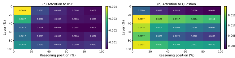
Figure 1: Qwen2.5-Math-7B에서 측정된 토큰별 어텐션 질량(suffix, MATH-500 500문제, 문제마다 독립 RSP). (a) RSP 토큰 어텐션은 추론 위치 축(가로)에서 감소하며, 이는 Theorem 1의 cache-growth 상계와 일치한다. 레이어 축(세로)의 추가 감소는 별도의 경험적 현상으로, 깊은 레이어에서 실제 토큰과 RSP 토큰 사이의 logit gap이 더 날카로워지는 경향을 시사하지만 Theorem 1만으로 직접 따라오지는 않는다. (b) 질문 토큰 어텐션은 비교적 균일하게 유지된다. 그림에 보고한 양은 Appendix F의 per-token mass로, RSP 길이 L 로 나눈 평균 값이며 본문 w_{r,i}^{(\ell)} 와는 상수배 관계다.
