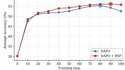
Figure 5: Qwen2.5-Math-7B의 7-벤치마크 평균 정확도. DAPO + RSP는 step 90에서 더 높은 peak에 도달하고 step 100까지 안정적으로 유지되는 반면, DAPO는 step 80 이후 감소한다.
