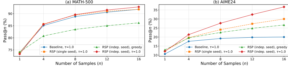
Figure 4: Qwen2.5-Math-1.5B-Instruct에서의 Pass@ N 스케일링. 좌측은 MATH-500, 우측은 AIME24이며, 문제당 N = 16 개의 샘플을 사용했다. Baseline은 temperature sampling만, fixed seed는 고정된 하나의 RSP와 temperature를 함께 쓴 경우, indep. seed는 샘플마다 다른 RSP를 쓰는 경우이다.
