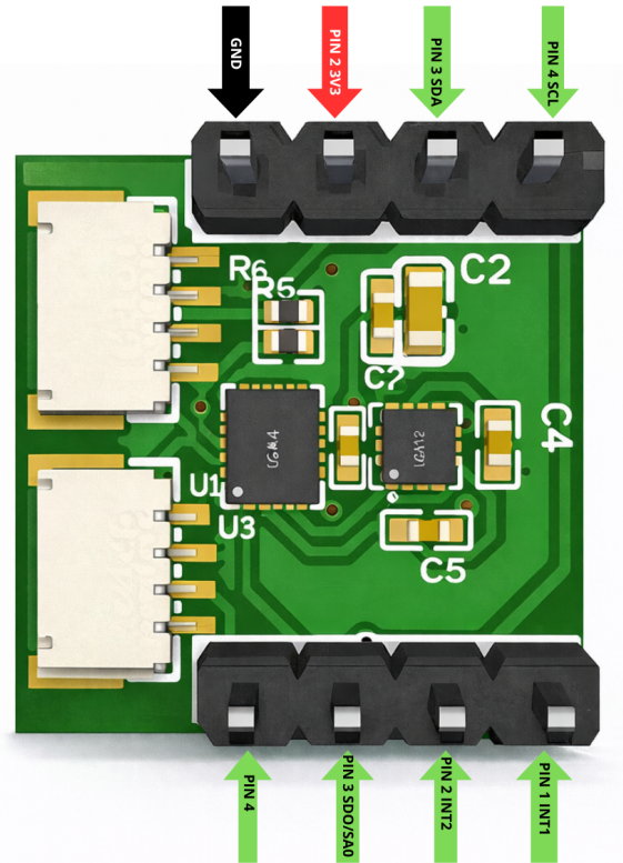
Figure 2: Diagrama de pines de la NOVA_sense
