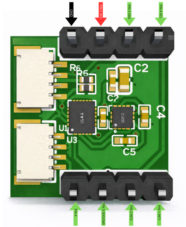
Figure 2: Diagrama de pines de la NOVA_sense
