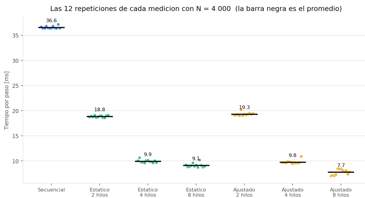
Figura 7. Las doce repeticiones de cada medicion con N = 4 000. Cada punto es una repeticion y la barra negra marca el promedio. La dispersion crece visiblemente al usar mas de cuatro hilos.
