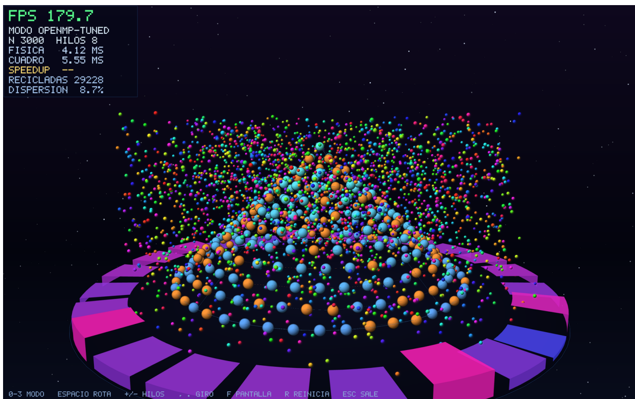
Figura 11. Configuración por omisión a pantalla completa (3024 x 1898): N = 3\,000 pelotas lloviendo sobre una piramide de 277 clavijas repartidas en 12 niveles, con 24 sectores contadores en la base, cuya altura y color crecen con la cantidad de pelotas que recibe cada uno. Las clavijas grandes en tonos frios forman la estructura; las ambar son las que oscilan. El fondo con degradado y campo de estrellas evita que el lienzo quede vacío: la escena ocupa la pantalla completa.
