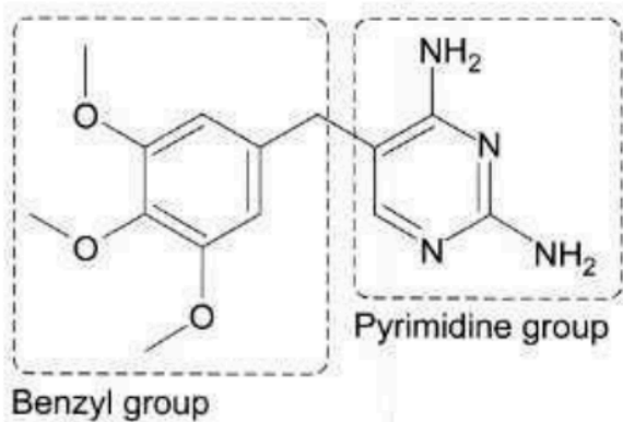
Trimethoprim
