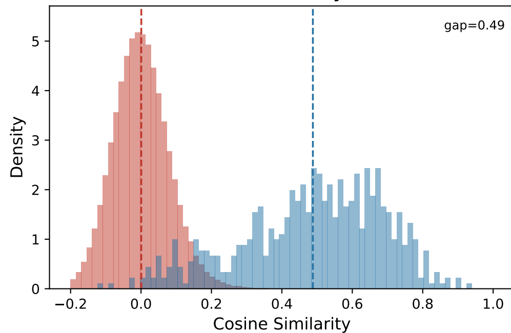
ABTT - Last Layer
