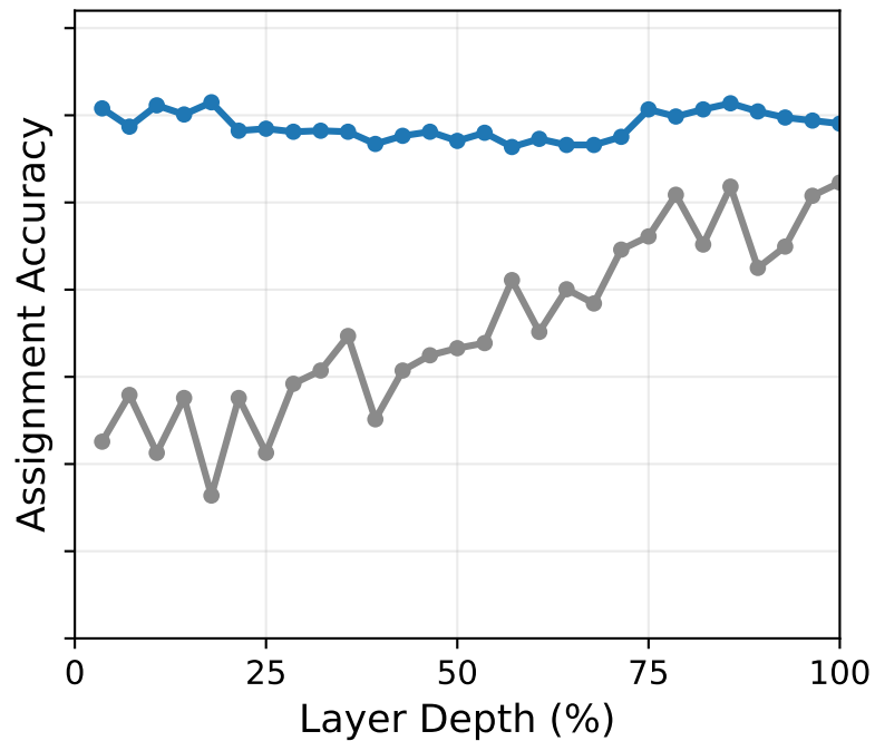
Qwen3-0.6B
