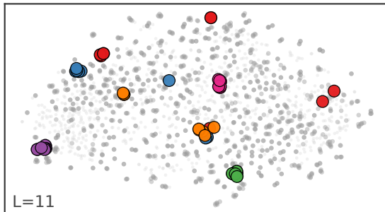
Baseline
