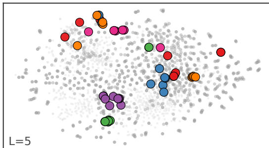
Qwen3-0.6B
