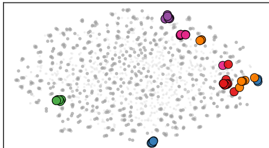
ABTT (D=10)
