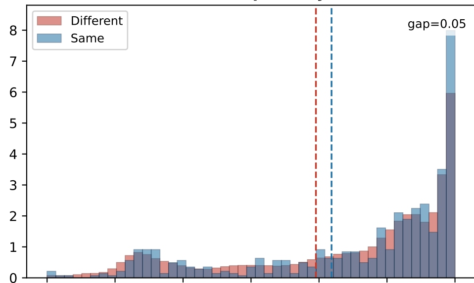
ABTT · Collapsed layer (L8)
