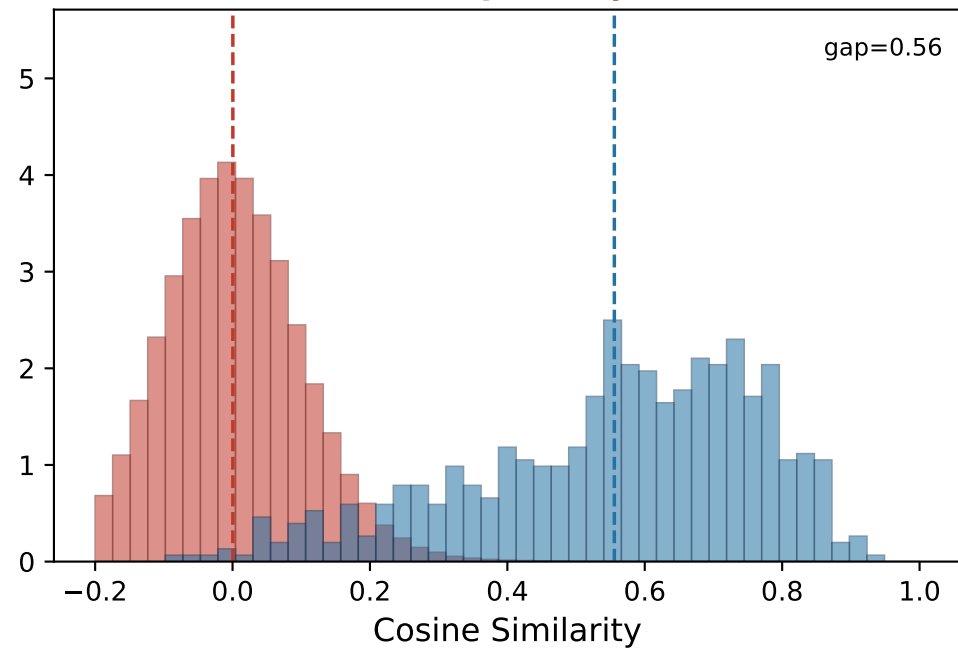
ABTT · Collapsed layer (L8)
