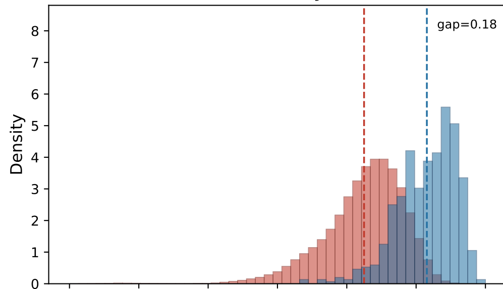
ABTT · Last layer (L12)
