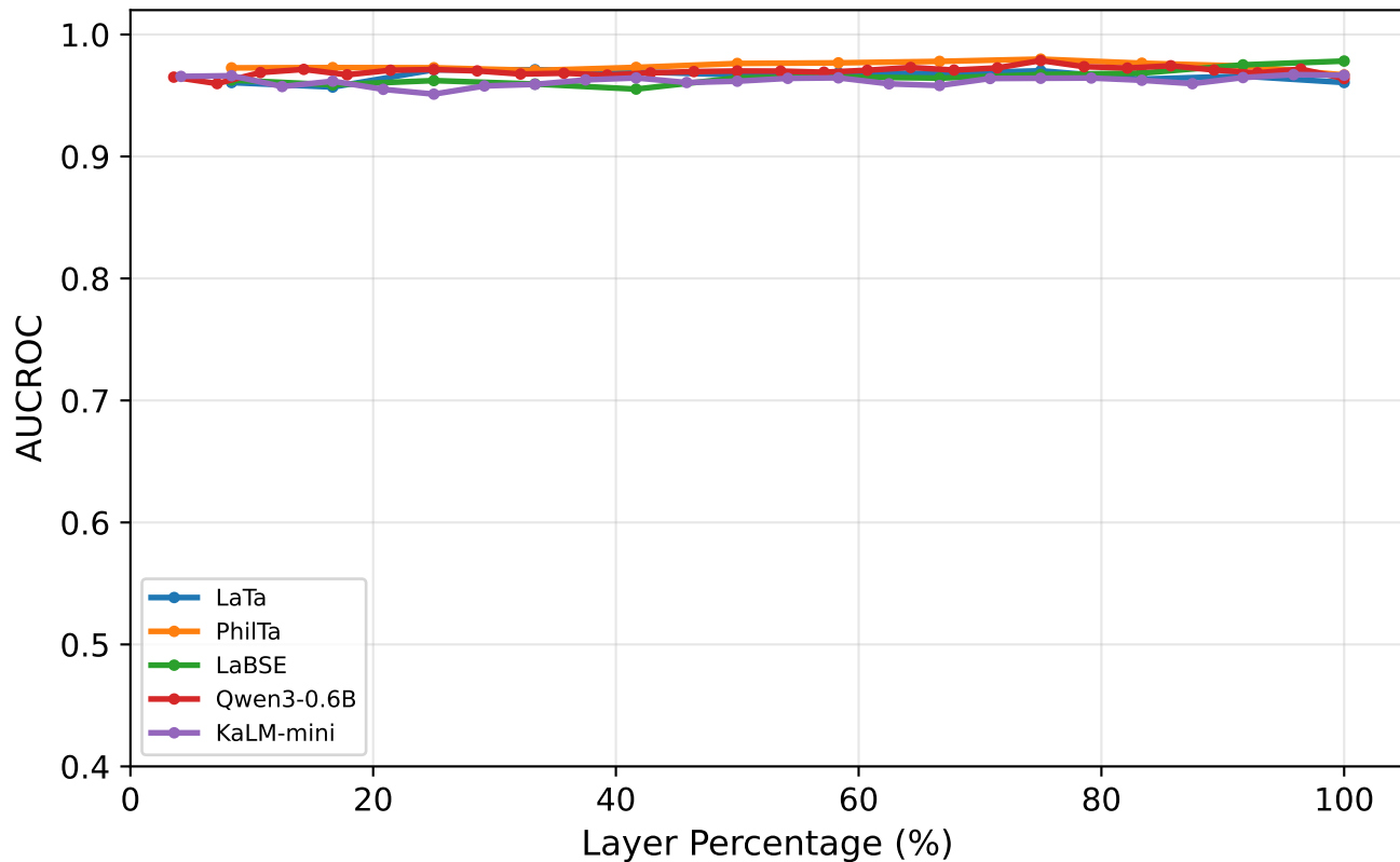
(A) AUCROC
